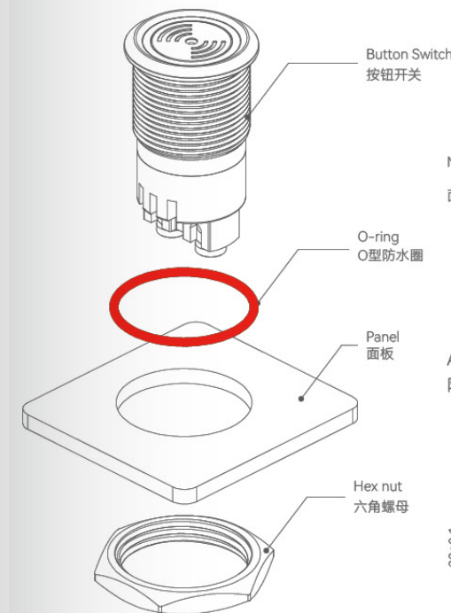
Installation method diagram 安装方式示意图
