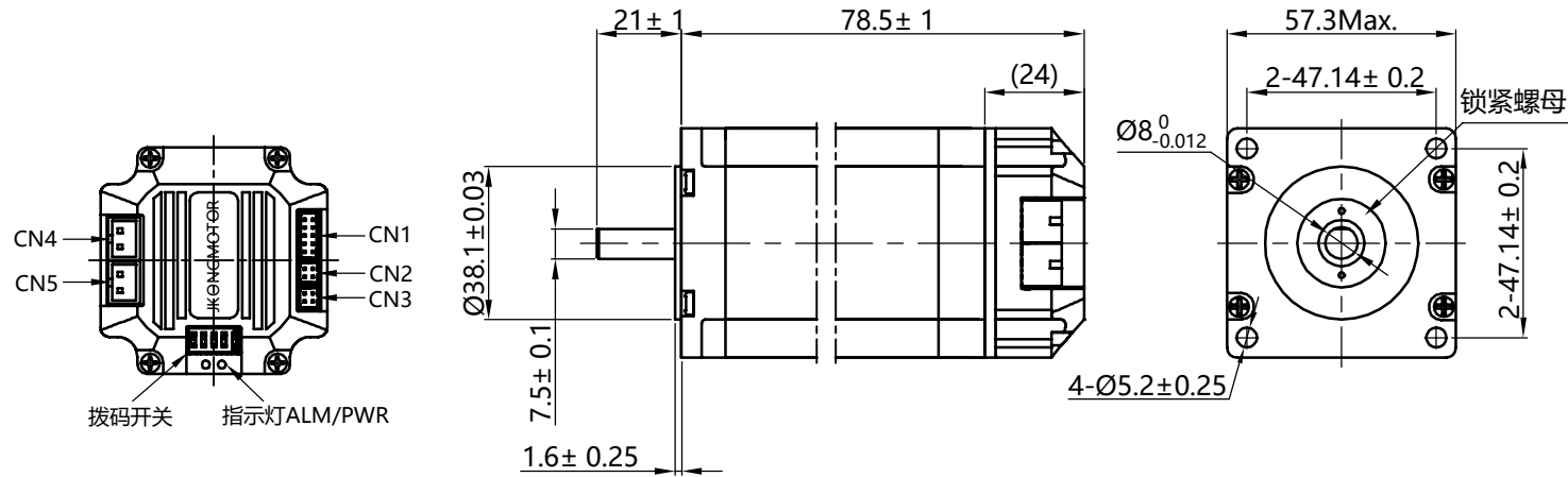
CN4 刹车电阻端口
